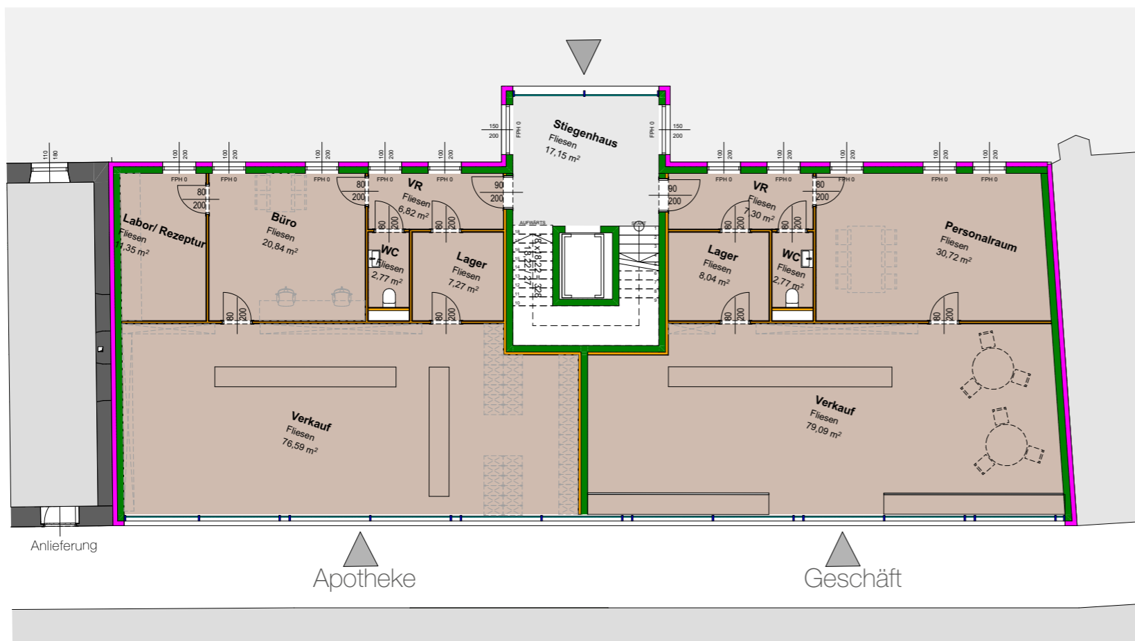
Erdgeschoss
