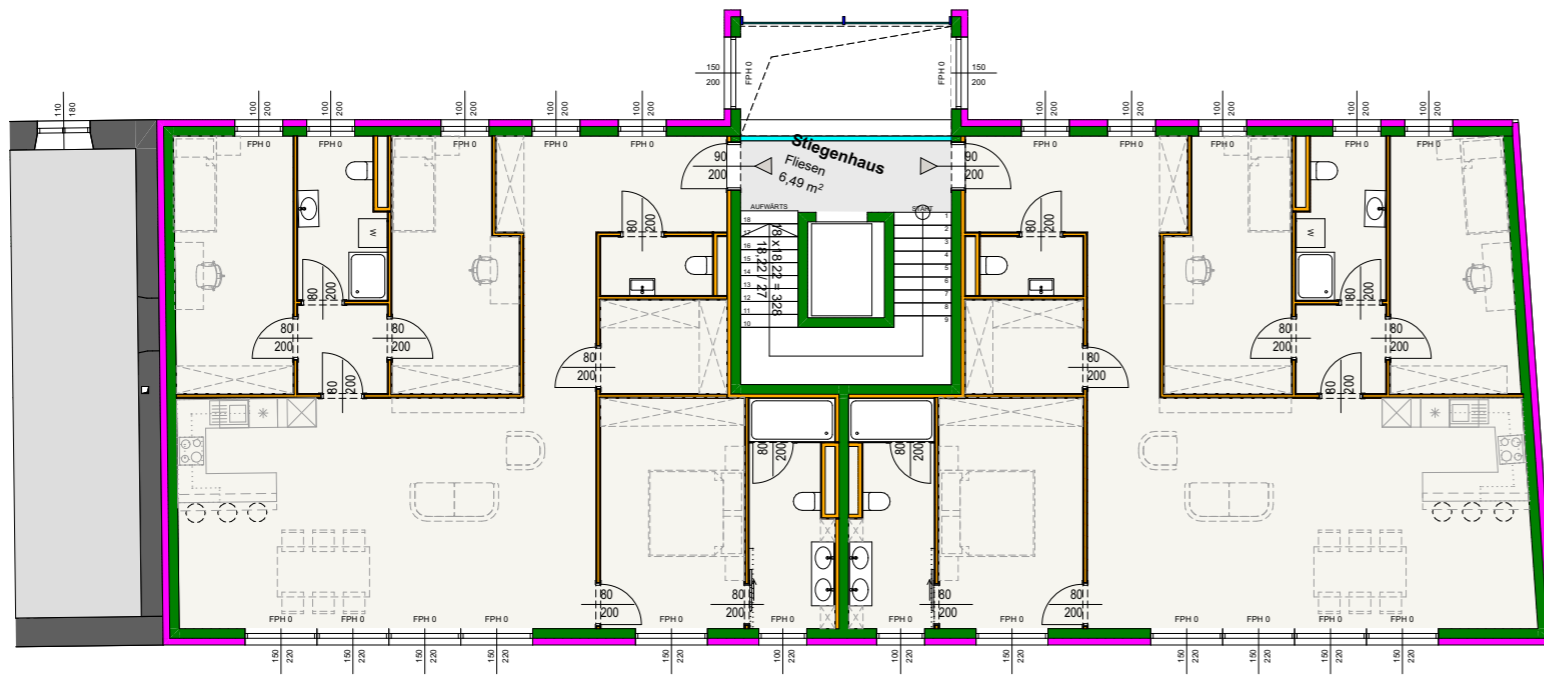
Obergeschoss
