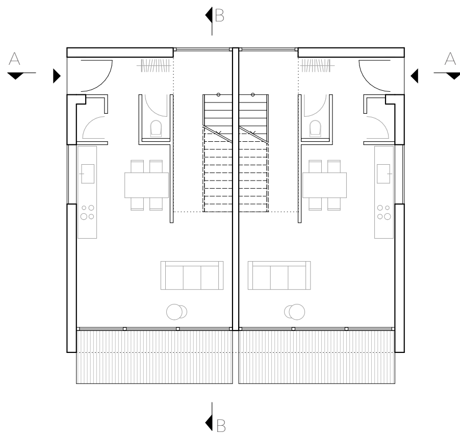
ERDGESCHOSS
