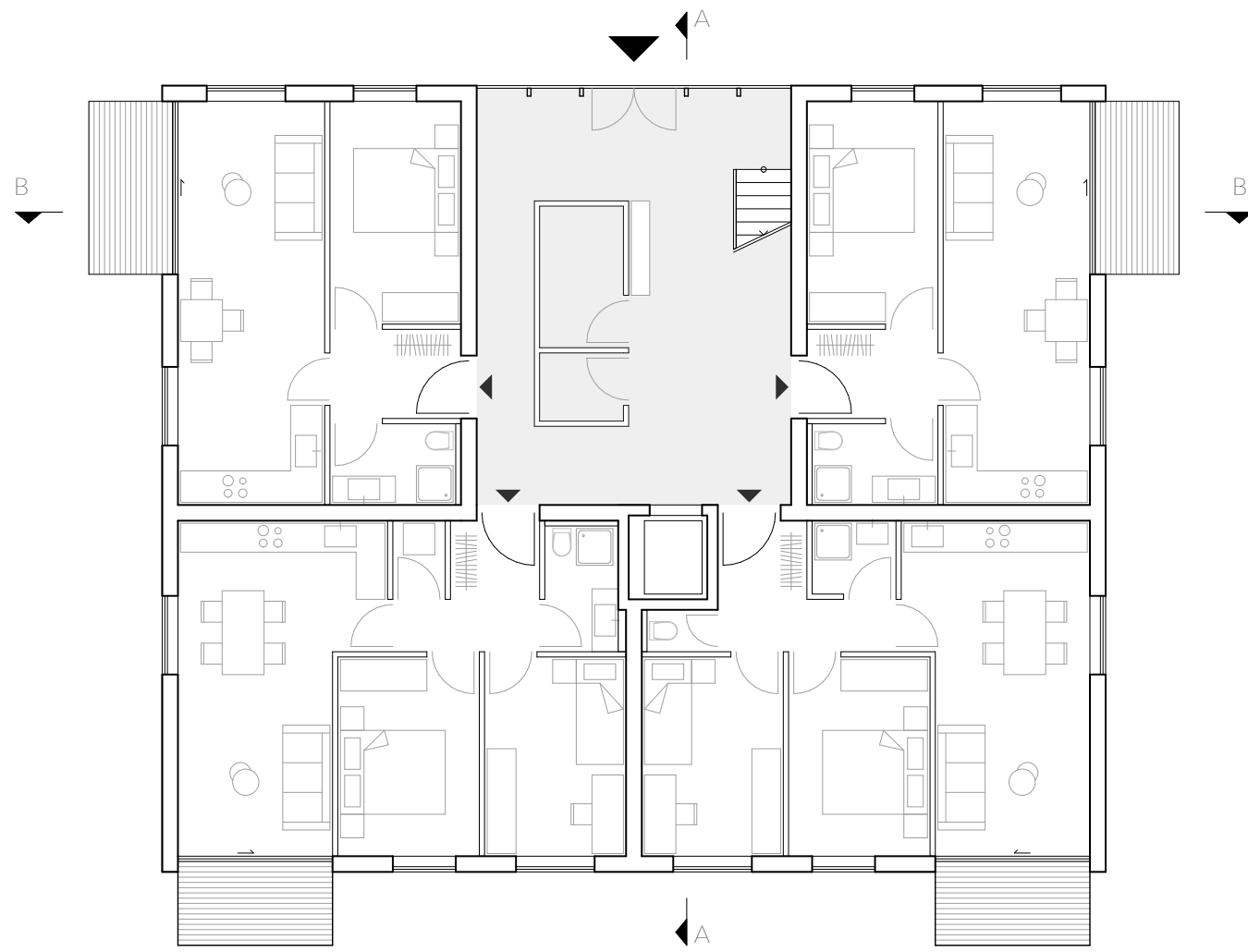
ERDGESCHOSS
