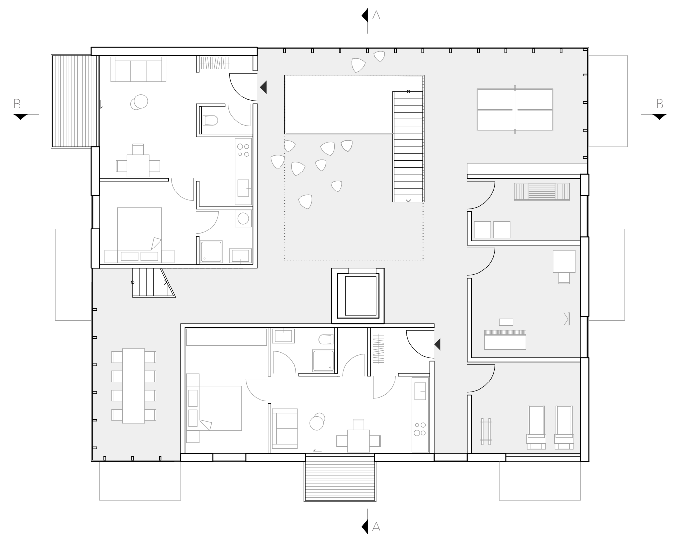
2. OBERGESCHOSS
