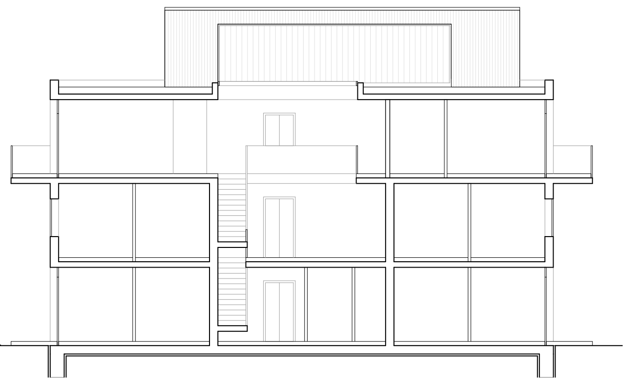
SCHNITT BB
