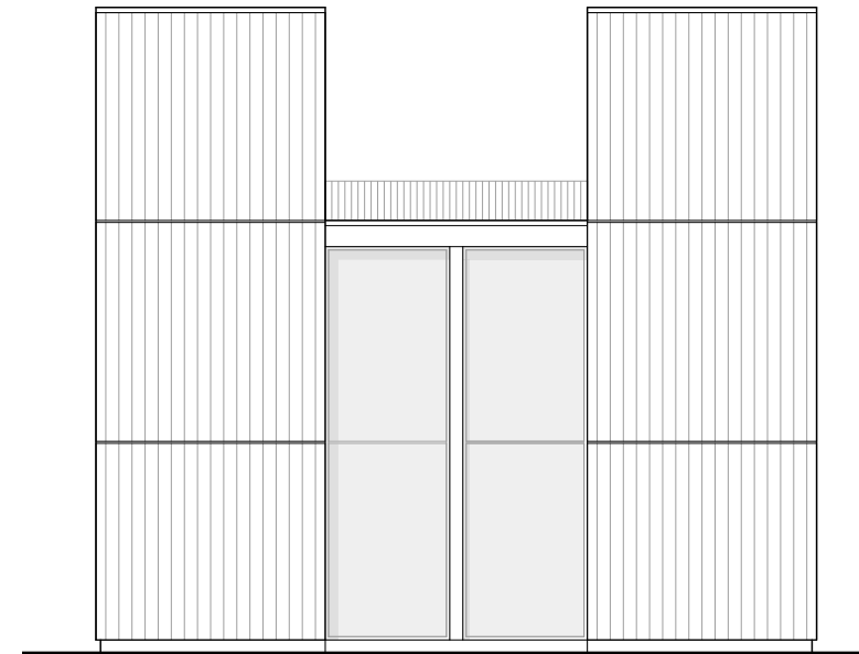
ANSICHT NORDOST
