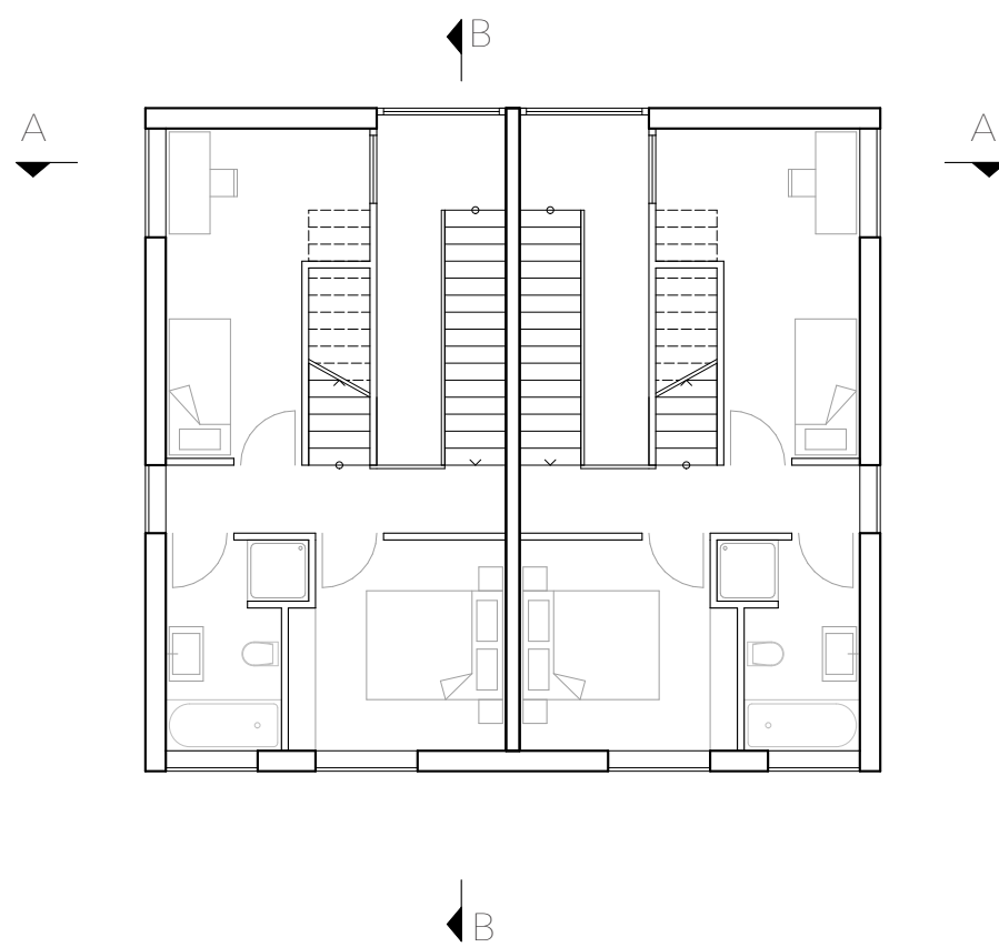
OBERGESCHOSS
