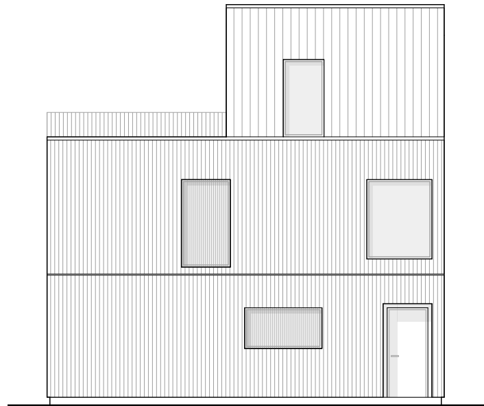
ANSICHT SÜDOST
