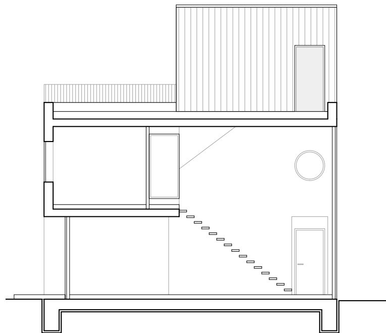
SCHNITT B-B
