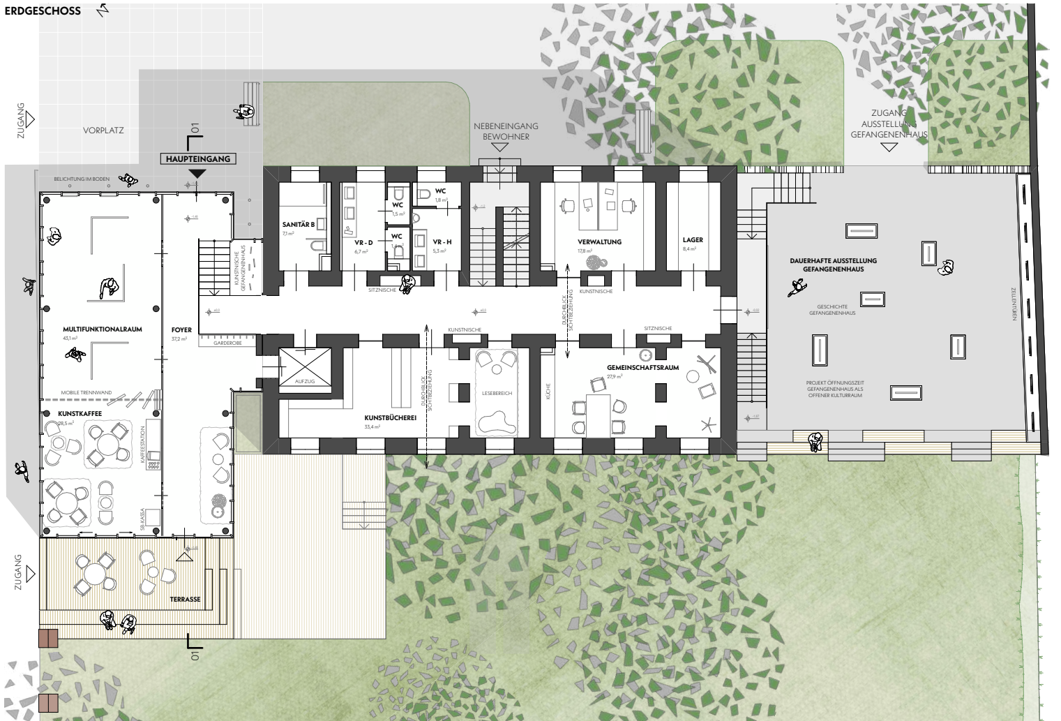
ERDGESCHOSS
