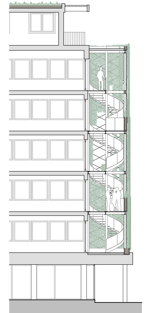
FASSADENSCHNITT Dachbegrünung
