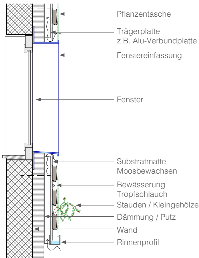
SYSTEMSCHNITT FASSADENBEGRÜNUNG Direktbewuchs Substratmatten
