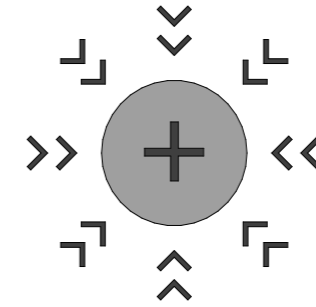
Attraktor
