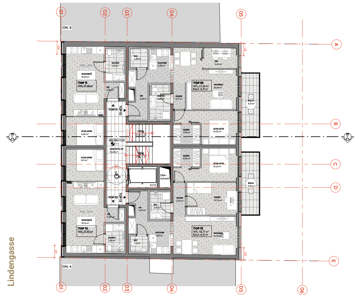
Grundriss 4. Obergeschoss
