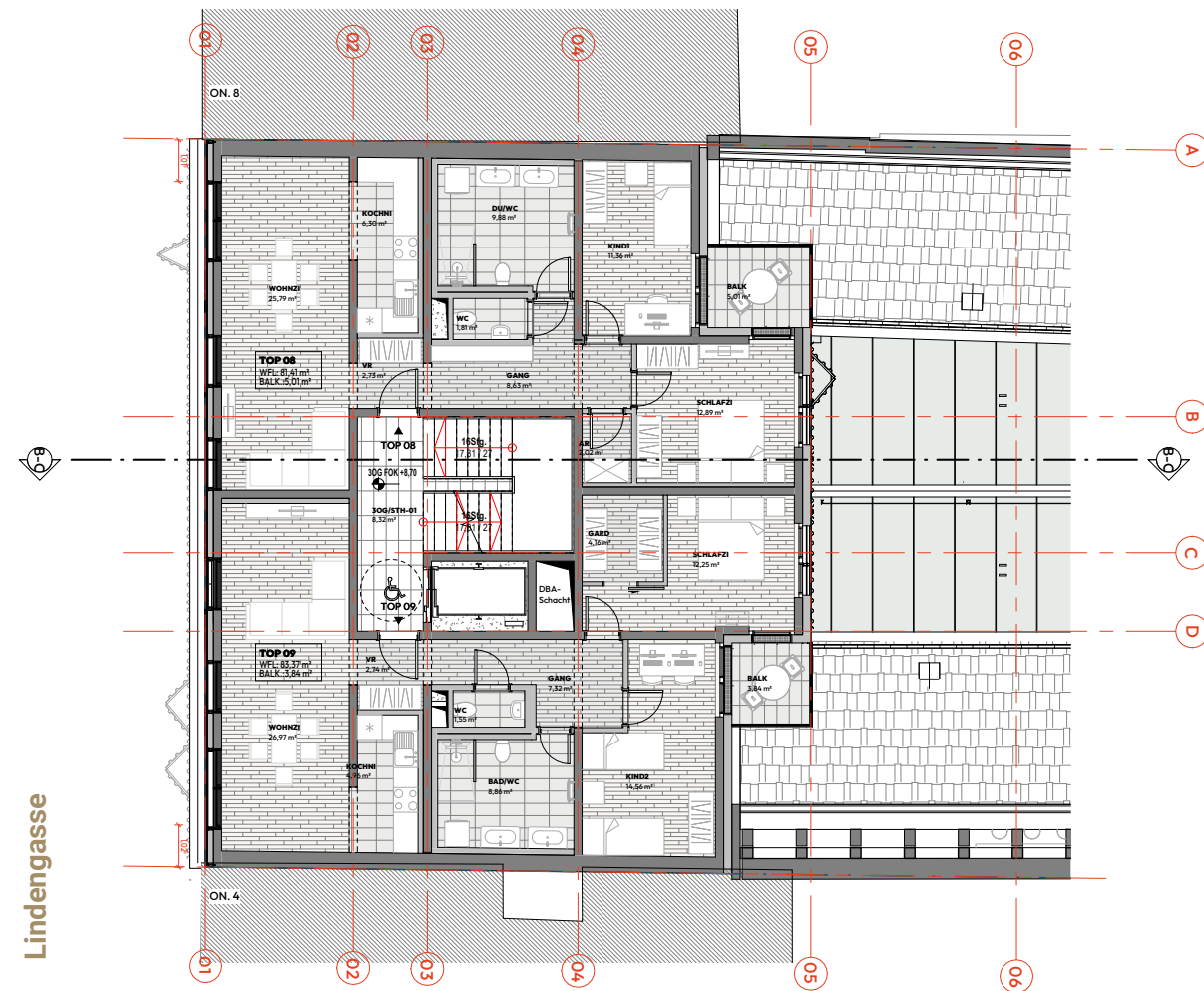
Grundriss 3. Obergeschoss
