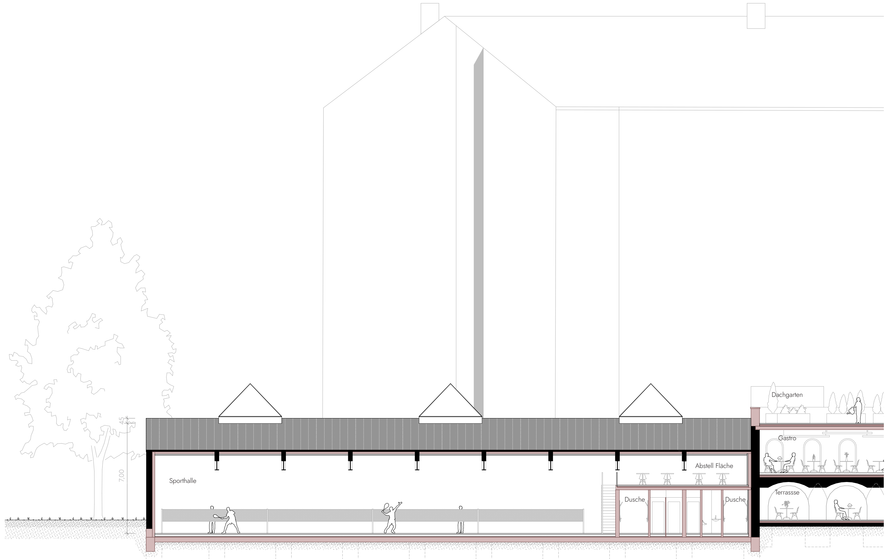
Schnitt A-A
